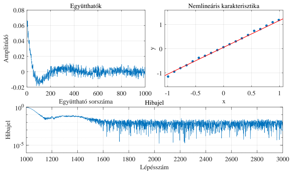
47. ábra. Shaker-identifikálása Hammerstein-modellel.
