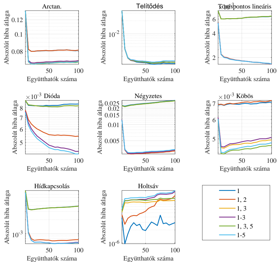
33. ábra. Volterra-modell hibajelének alakulása különbéféle hatványok és együtthatószám esetén, LMS algoritmussal
