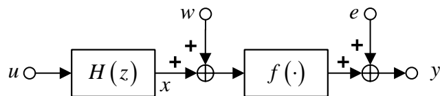
14. ábra. Wiener-modell folyamatot és mérést terhelő zajjal. [30] alapján.
