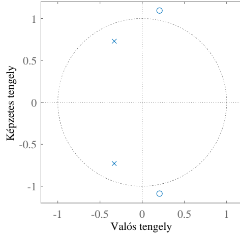
29. ábra. A H(z) rendszer pólus-zérus térképe.
