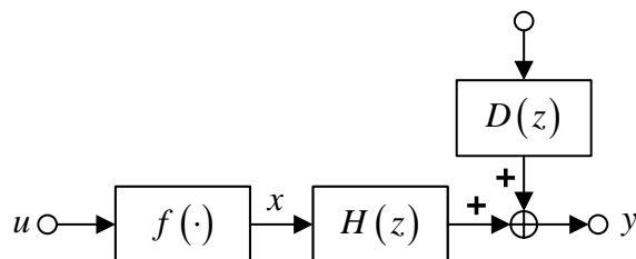
13. ábra. A Hammerstein-modell szűrt zajjal. [31] és [1] alapján.
