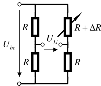
18. ábra. Hídkapcsolás.
