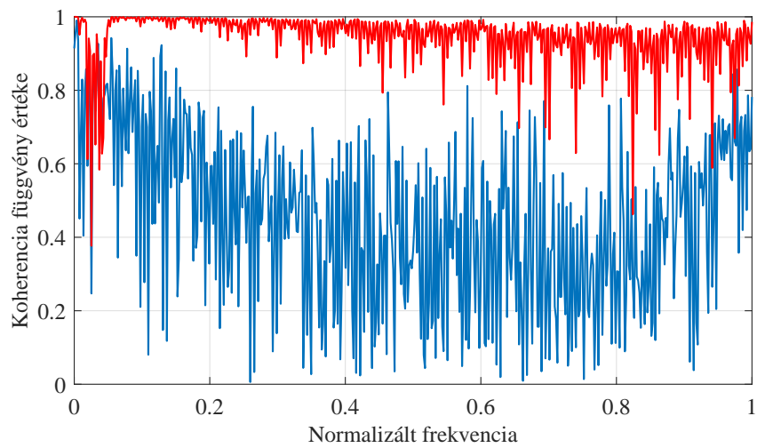
43. ábra. A shaker Volterra-moddal kompenzált és nem kompenzált kimenetének koherenciafüggvénye
