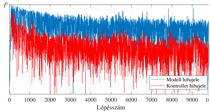
35. ábra. XLMS algoritmus offline modelljének és az online adaptált kontrollerének hibajele.
