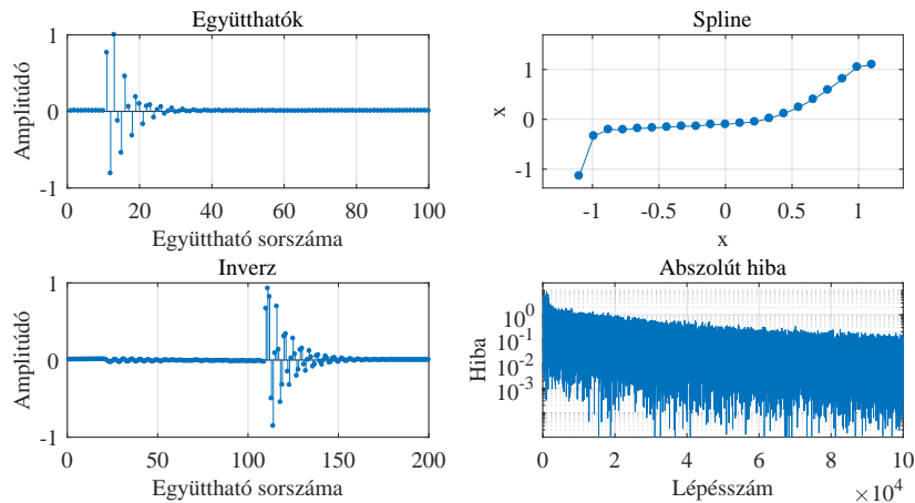
44. ábra. Diódát tartalmazó rendszer identifikálása
