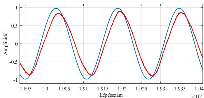
38. ábra. Shaker gerjesztése és kimeneti jele.
