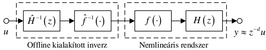
2. ábra. Nemlineáris rendszer kompenzálása offline meghatározott inverzzel
