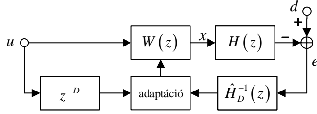
23. ábra. Az ELMS algoritmus. [15] alapján.
