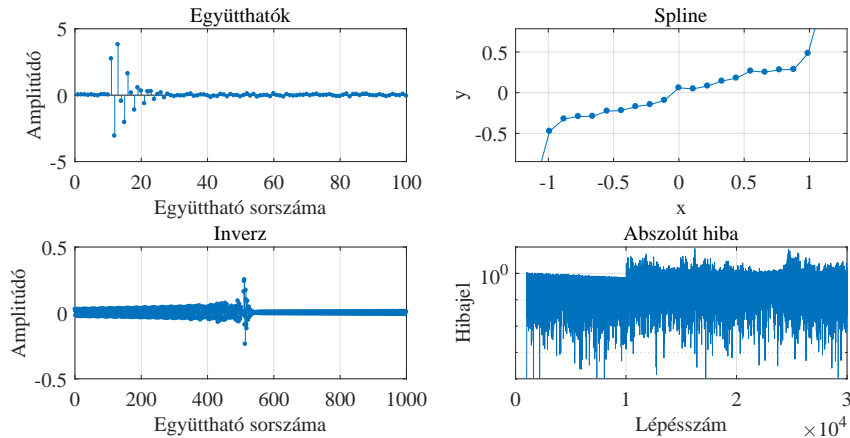
46. ábra. Wiener-modell alapú, arctan függvényt tartalmazó rendszer Hammerstein-moddal történő identifikálásának eredménye.
