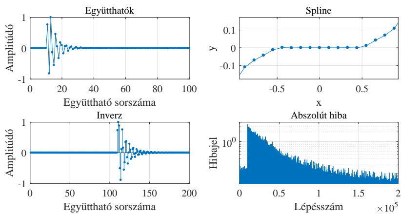
45. ábra. Holsávot tartalmazó Hammerstein-modell
