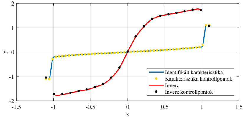
50. ábra. Identifikált spline függvény és inverze.
