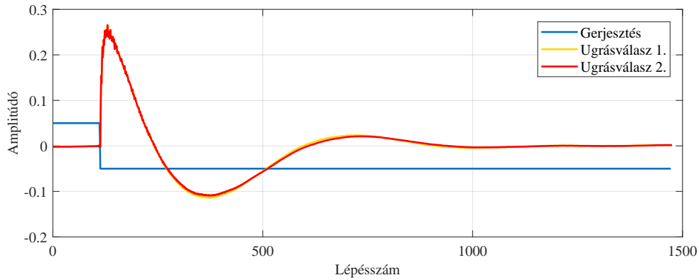
39. ábra. A shaker ugrásválasza
