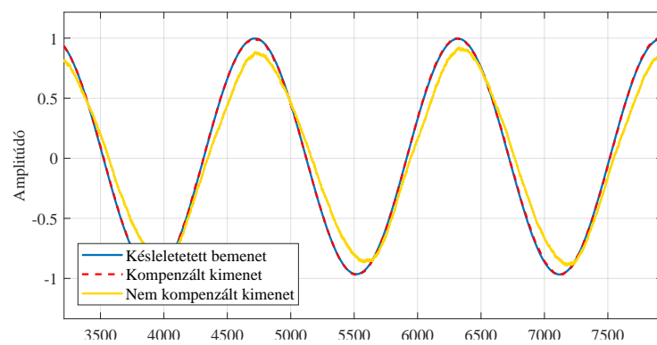
42. ábra. Shaker késleletett gerjesztése, kompenzált és nem kompenzált kimenete.
