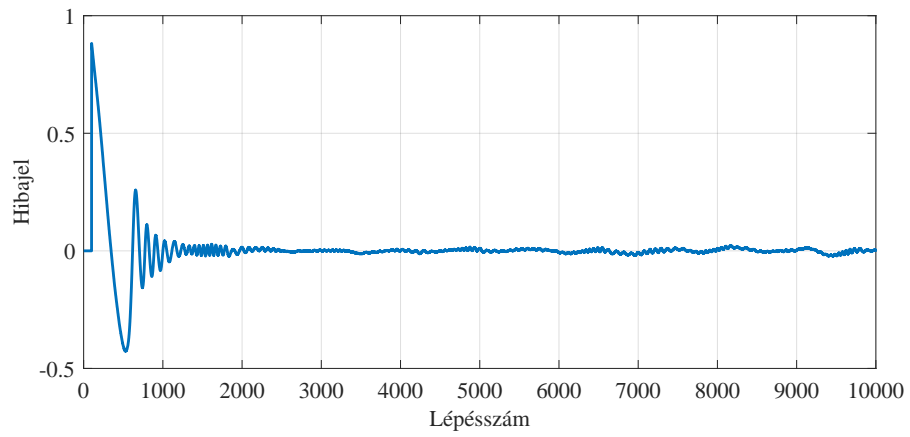
41. ábra. Controller hibajele shaker kompenzálásakor.
