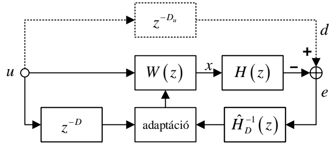
24. ábra. Az ELMS algoritmus kompenzálásra használható módosítása.
