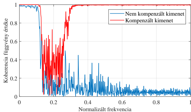
37. ábra. Volterra-modellel kompenzált és kompenzálatlan rendszer kimenetének koherenciafüggvénye arctan-szerű karakterisztikánál és szűrt bemenő zaj gerjesztésnél.
