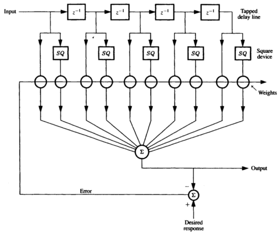
7. ábra. Egyszerűsített Volterra-modell blokkvázlata.
