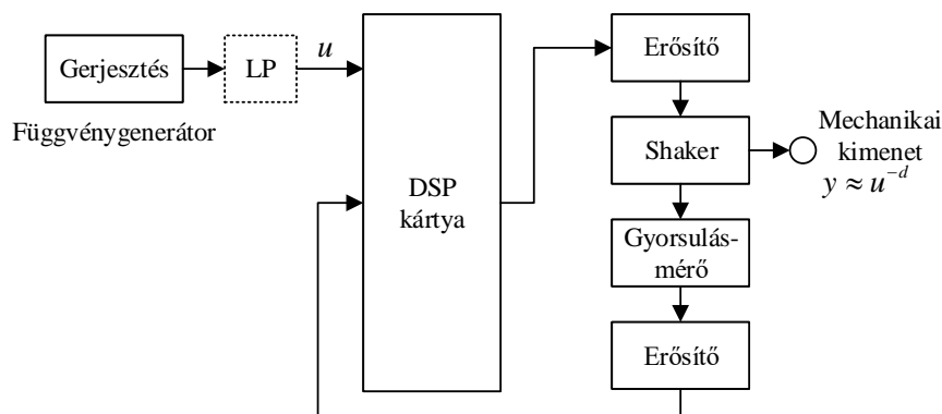
53. ábra. Shaker DSP kártyával történő kompenzálás
